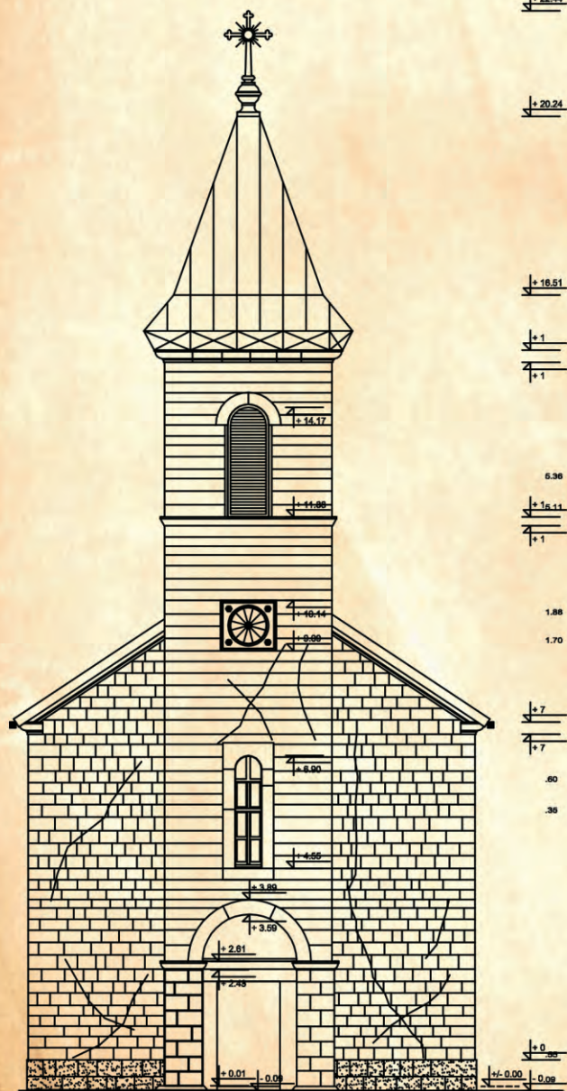
Западна фасада
