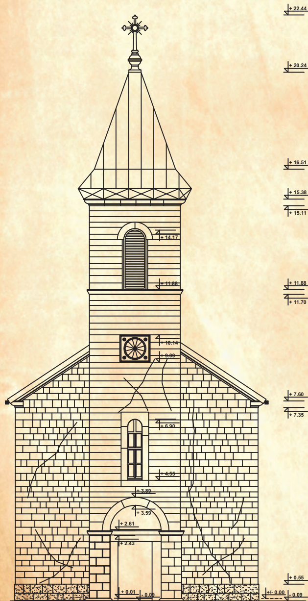
Западна фасада
